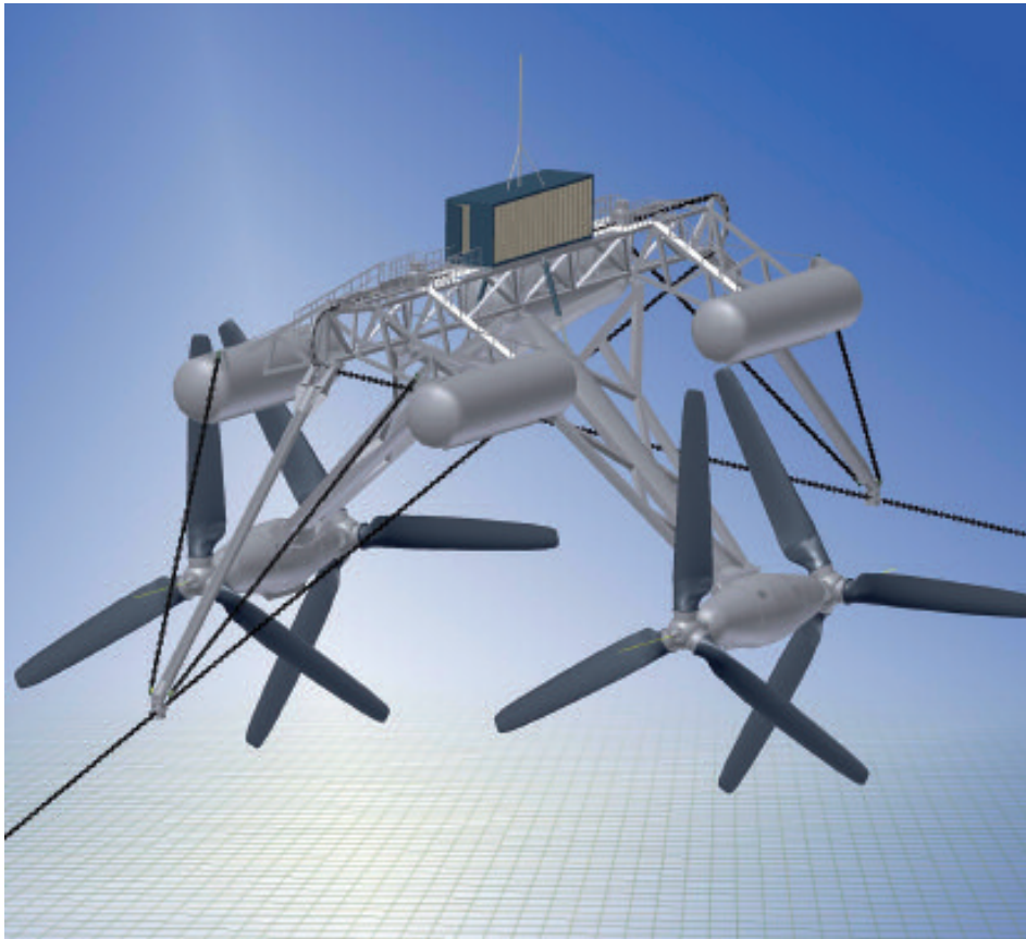
Figur 7.4 Tidevannsenergiverk
