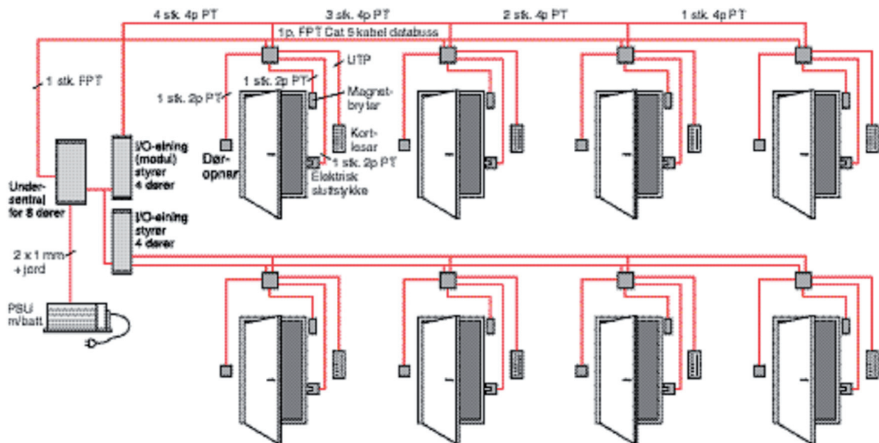
Figur 5.6 Adgangskontrollanlegg (Siemens-Cerberus)
