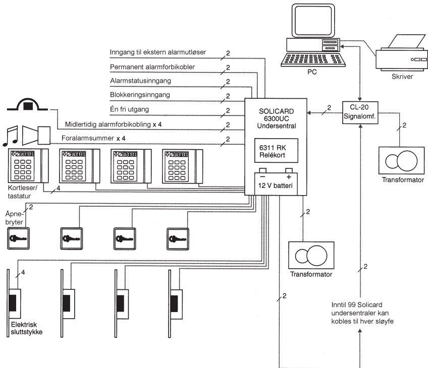
Figur 5.1 Et system for adgangskontroll
