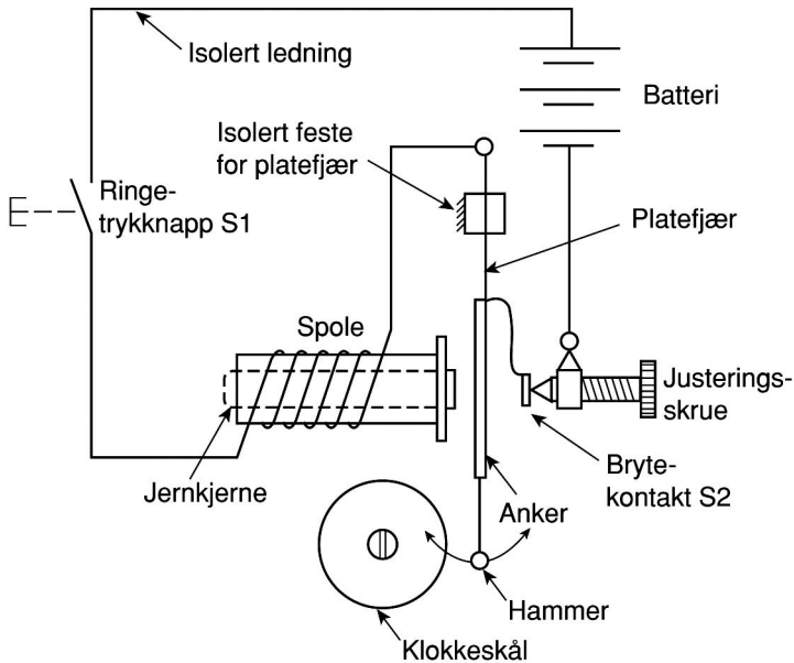
Figur 2.4 Prinsippskisse for et ringeanlegg for likestrøm
