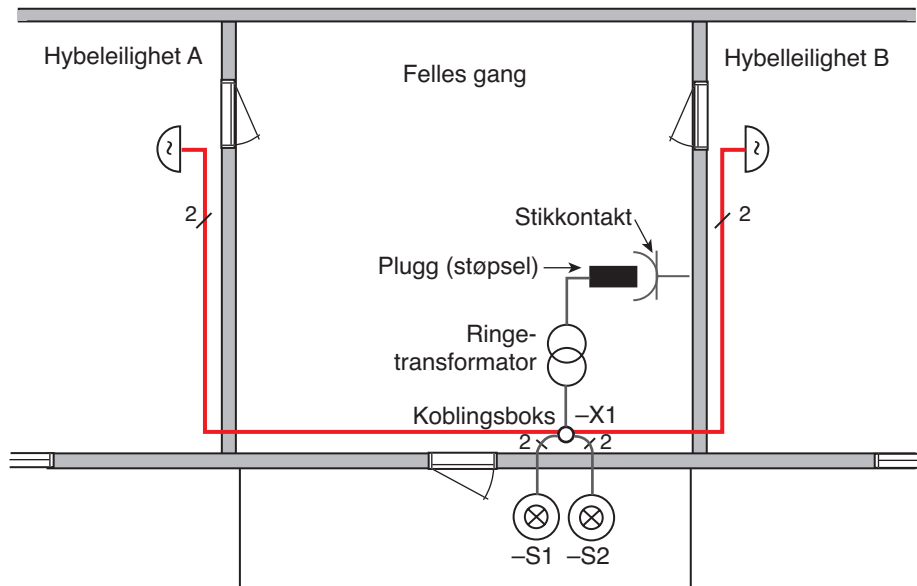
Figur 2.24 Installasjonstegning for ringeanlegget
