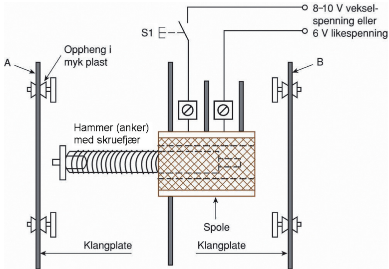
Figur 2.12 Klangklokke med to klangplater
