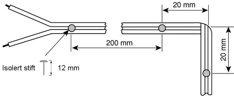
Figur 2.13 Festing av ringeledning
