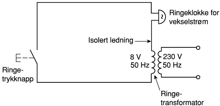
Figur 2.3 Strømkrets for vekselstrømsringeanlegg
