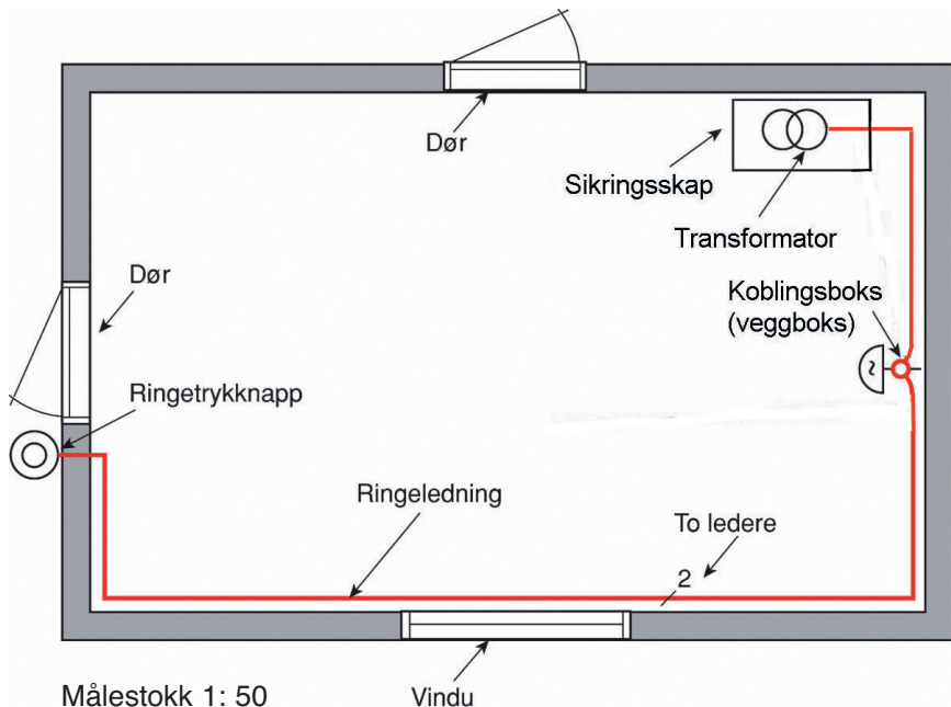
Figur 2.22 Åpen installasjon
