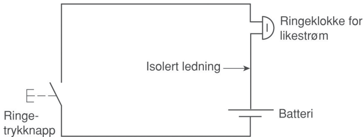
Figur 2.2 Strømkrets for likestrømsringeanlegg
