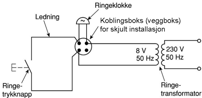
Figur 2.20 Koblingsskjema
