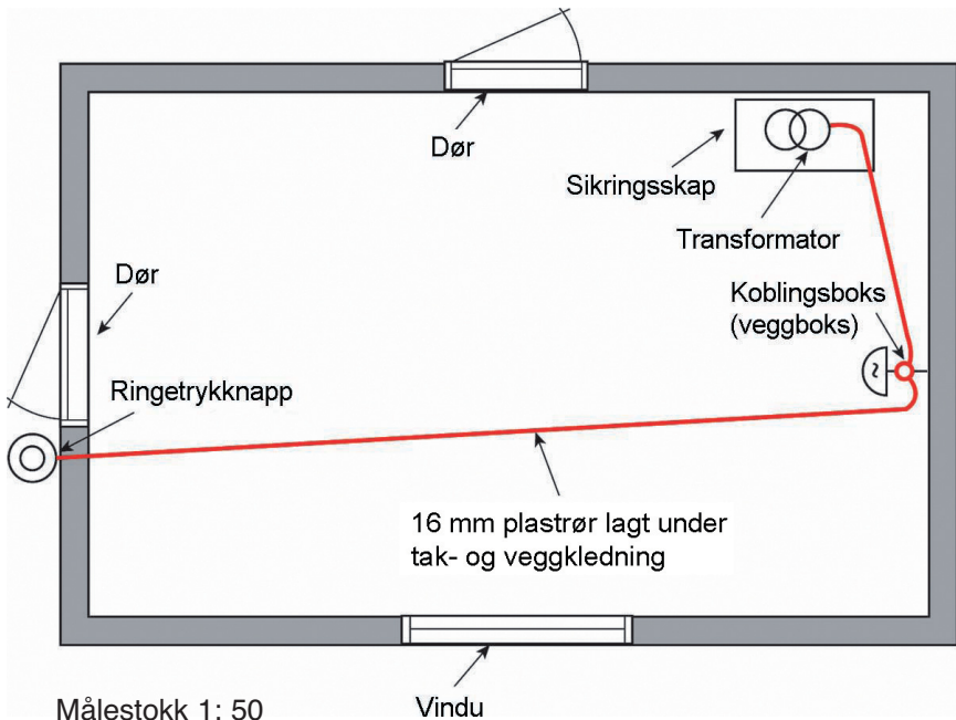
Figur 2.23 Skjult installasjon
