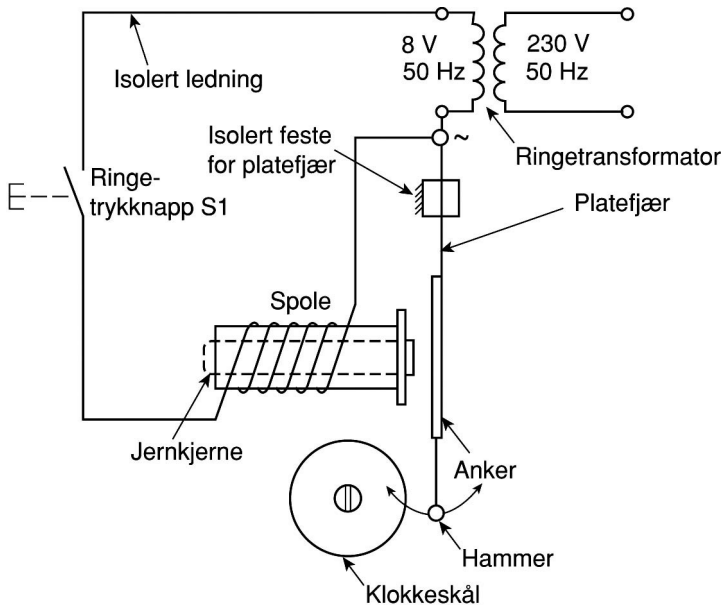
Figur 2.5 Prinsippskisse for et ringeanlegg for vekselstrøm
