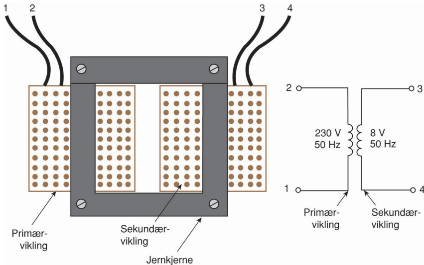
Figur 2.6 Skisse og koblingsskjema for en ringtransformator
