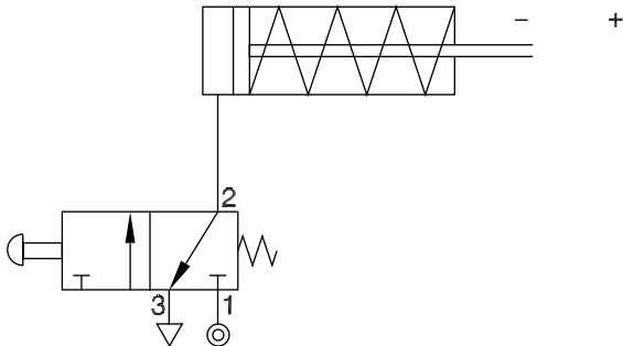
Figur 15.9 Pneumatisk koblingskjema for styring av en enkeltvirkende sylinder med manuelt aktivert 3/2 ventil
