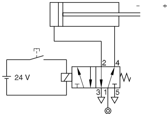
Figur 15.11 Elektropneumatisk koblingskjema for elektrisk styring av en dobbeltvirkende sylinder
