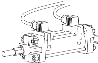
Figur 15.7 Sylinder med magnetstempel og magnetbrytere monteret utenpå cylinderrøret
