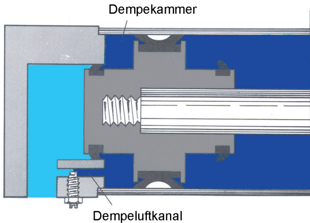
Figur 15.6 Luftdemping av stempelbevegelsen
