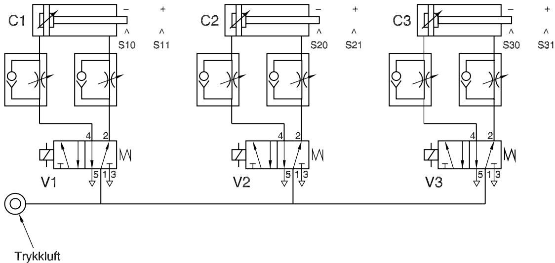
Figur 15.17 Pneumatisk koblingskjema for anlegget
