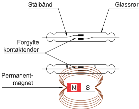
Figur 15.8 Prinsippet for en magnetkontakt
