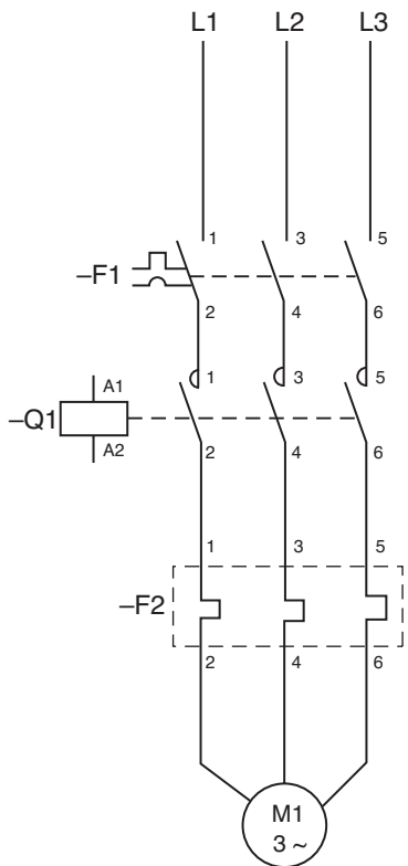
Figur 15.19 Hovedstrøms- og styrestrømsskjema
