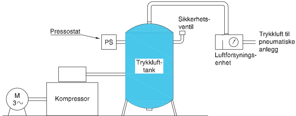
Figur 15.1 Prinsippskisse av et trykkluftanlegg
