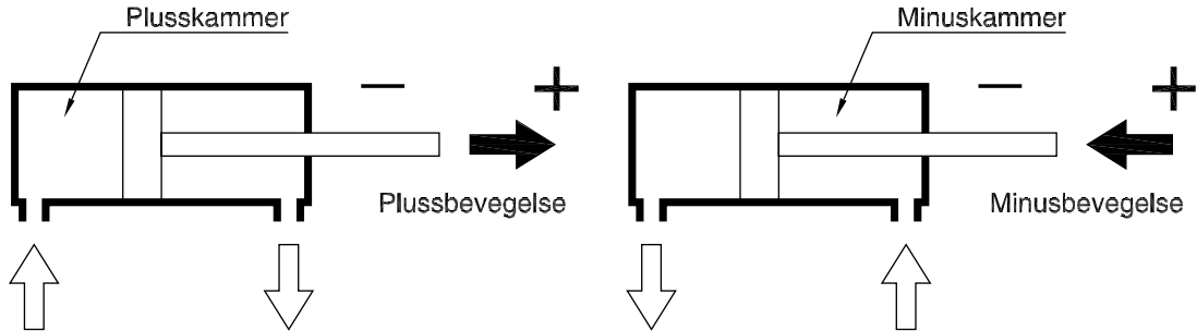
Figur 15.4 Pluss- og minuskammer og stempelbevegelsen til en dobbeltvirkende sylinder
