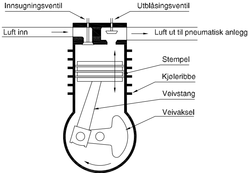
Figur 15.2 Prinsippskisse av en stempelkompressor
