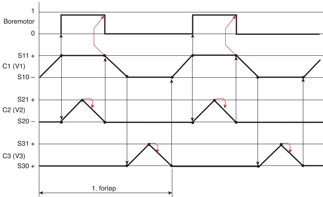
Figur 15.18 Forløpsdiagram for sylinderbevegelesene
