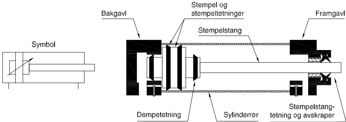
Figur 15.3 Dobbeltvirkende sylindere med endedempning
