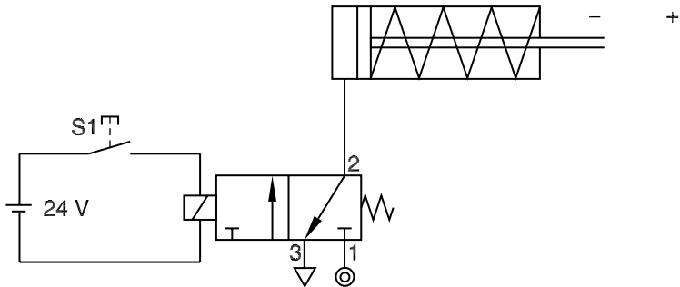
Figur 15.10 Pneumatisk koblingskjema for elektrisk styring av en enkeltvirkende sylinder.
