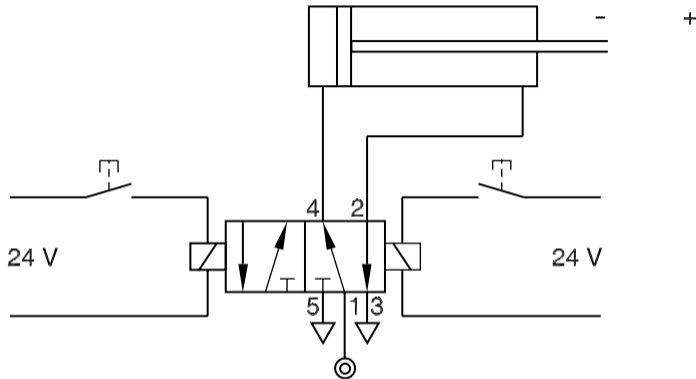
Figur 15.12 Pneumatisk koblingskjema for elektrisk styring av en dobbeltvirkende sylinder med bistabil retningsventil
