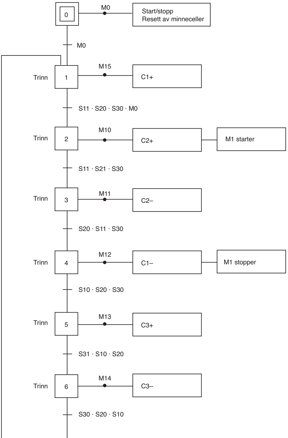
Figur 15.21 Sekvensielt funksjonsdiagram
