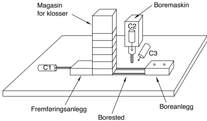
Figur 15.16 Benkeboremaskinen og konstruksjonsskissen for boreoperasjonen
