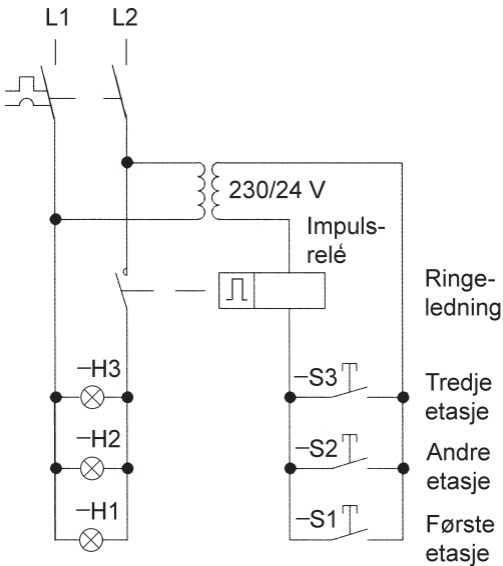
Figur 8.3 Lysstyring med impulsrelé
