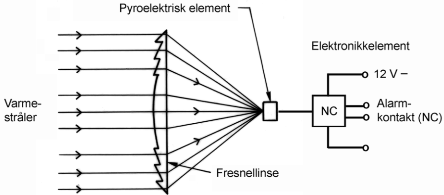
Figur 8.4 Blokkskjema for en PIR-detektor
