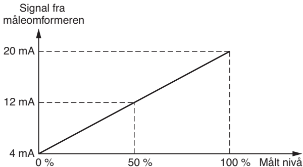
Figur 9.3 Forholdet mellom målt nivå i tanken og det elektriske signalet fra måleomformeren
