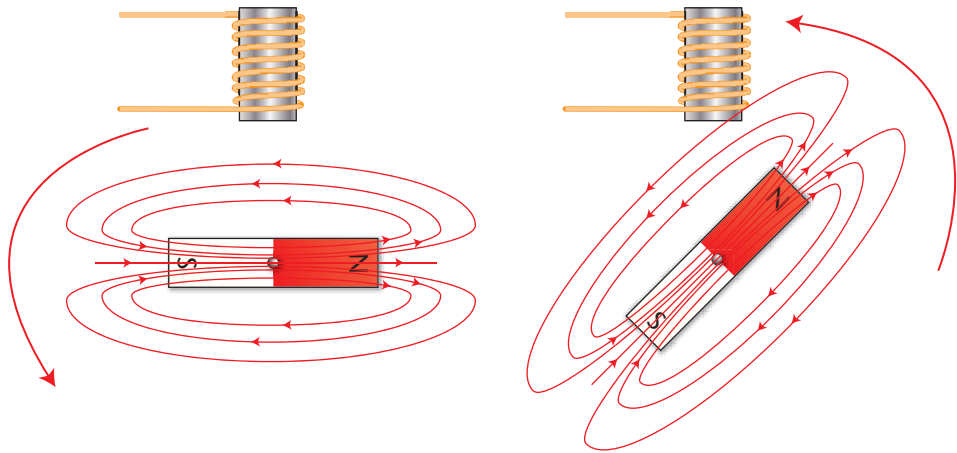
Figur 7.11 Generatormodell
