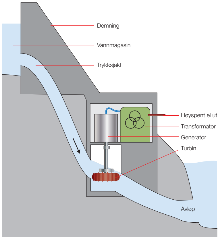
Figur 7.3 Vannenergiwerk
