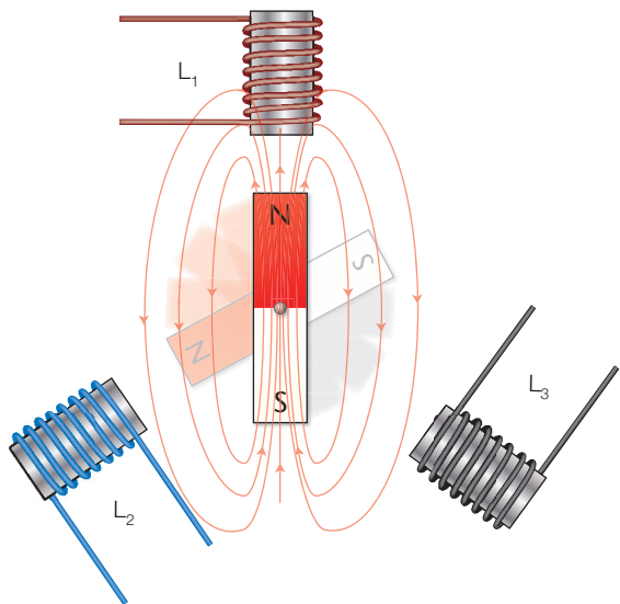
Figur 7.13 Trefaset generatorprinsipp
