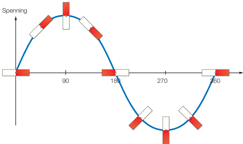
Figur 7.12 Sinuskurve
