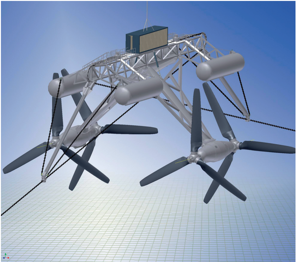
Figur 7.5 Tidevannsenergiverk
