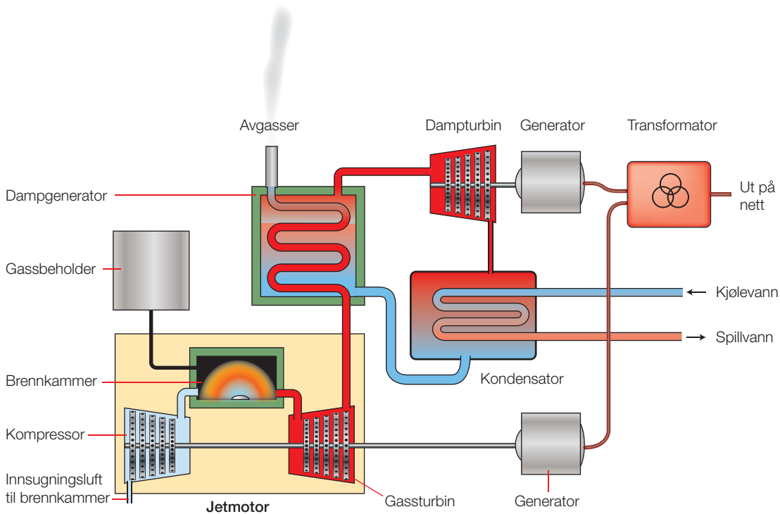
Figur 7.8 Gassmotorverk
