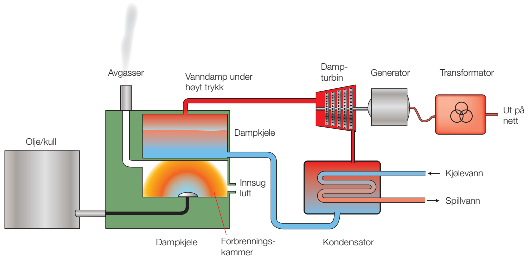
Figur 7.7 Varmeenergiverk
