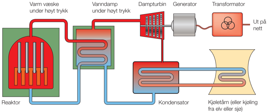
Figur 7.9 Kjerneenergiverk
